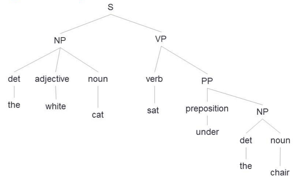
Parsing
