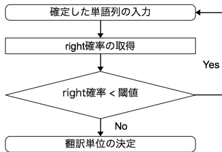
図3 翻訳単位の調整
