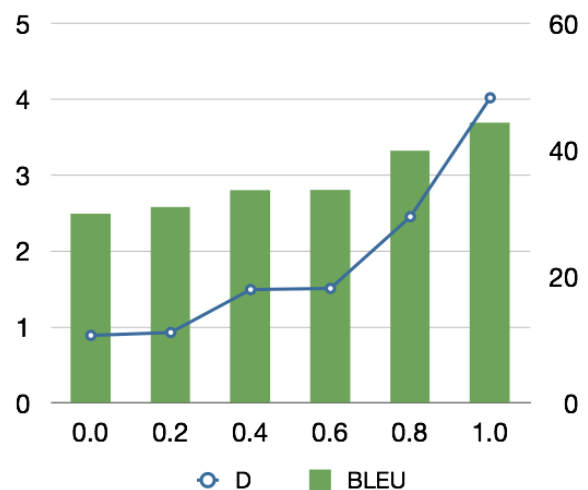
図 5 実験結果 (11 形態素以上)
