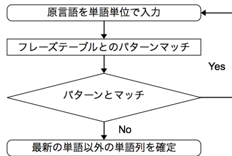
図 1 フレーズテーブルによる翻訳単位の決定
