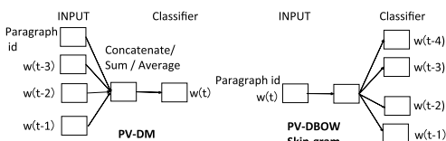
図 2 パラグラフベクトルの 2 種類のモデル Fig. 2 Two types of models for learning paragraph vectors.
