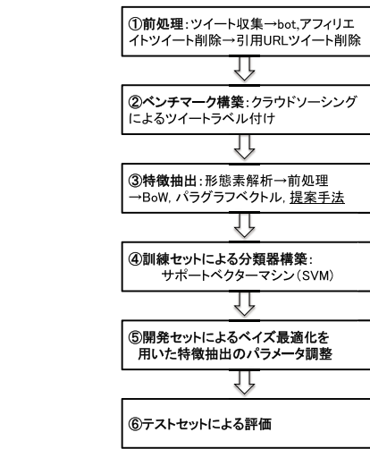
図 4 Twitter からの評判情報抽出の実験手順
