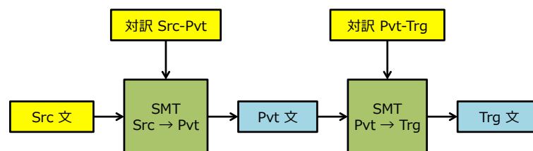
図 4 逐次的ピボット翻訳
