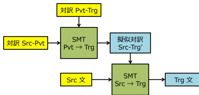
図 5 擬似対訳コーパス手法
