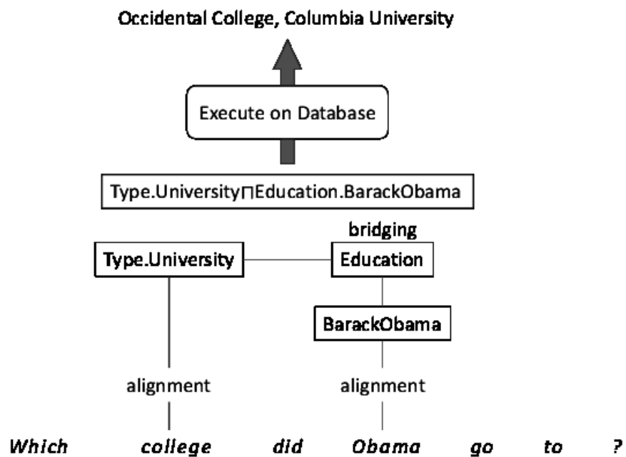
図 3 SEMPRE フレームワークによる質問応答の動作例
